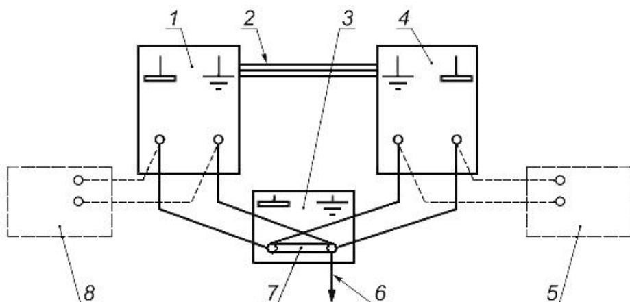
Рисунок 3 - Схема подачи кратковременных посылок тока на цепи защитного и сигнального заземления испытуемого ТС АС (вариант 1)
