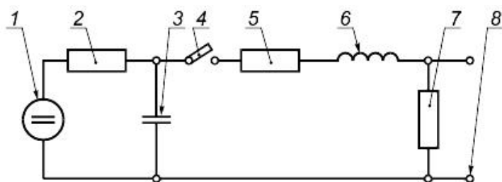
Рисунок 5 - Упрощенная схема ИГ токов микросекундных импульсных помех
