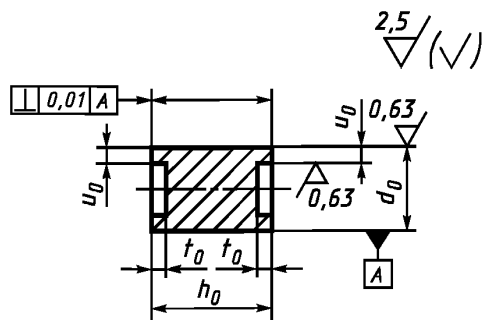
Рисунок 2 — Экспериментальные образцы IV типа
