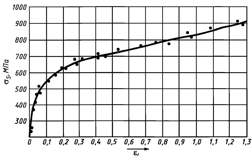
Рисунок 9 — Экспериментальная кривая упрочнения в координатах \sigma_s - \epsilon_l
