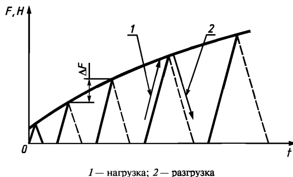
Рисунок 11 — Проведение испытаний при ступенчатом увеличении нагрузки
