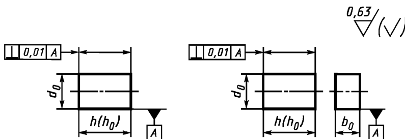
Рисунок 1 — Экспериментальные образцы I—III типов
