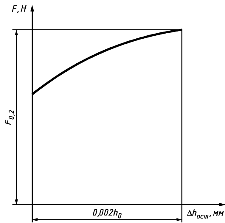
\Delta h_{ост} — абсолютная остаточная деформация (укорочение) образца
